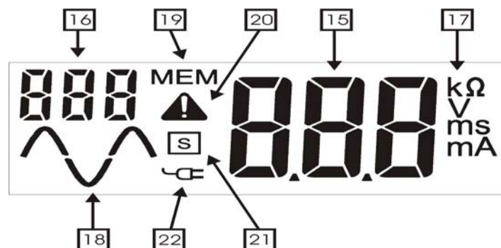
Рис.2. Жидкокристаллический дисплей прибора MIE-500.
